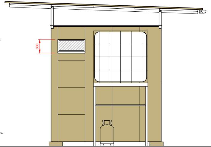
End Elevation
