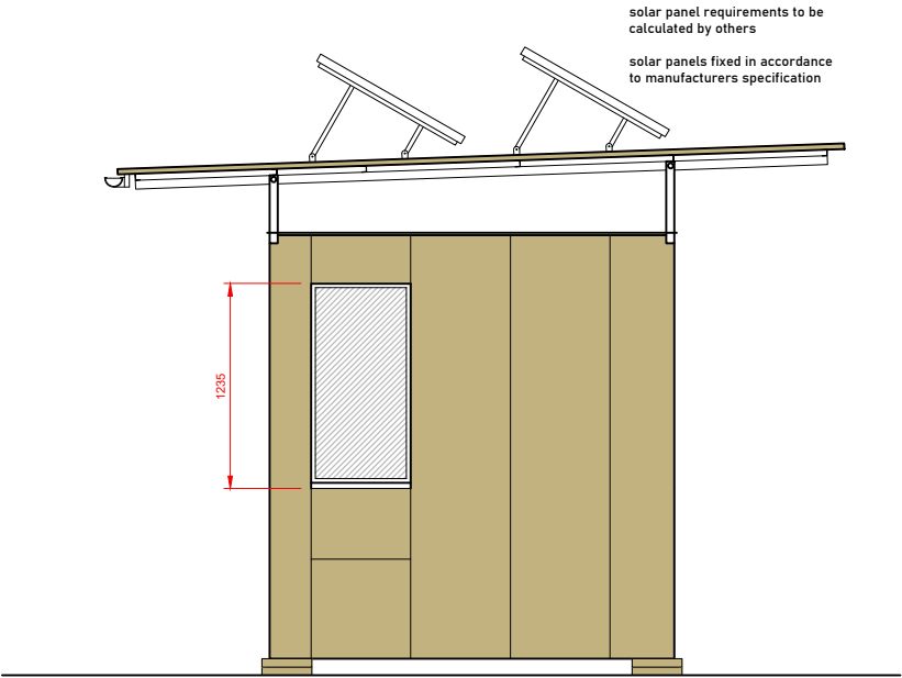
End Elevation
